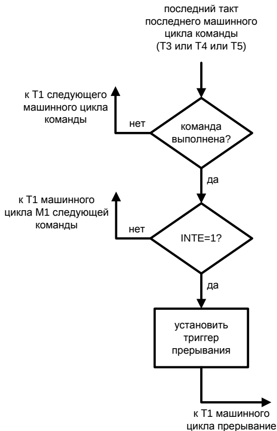
Рис. 66. Последовательность перехода в режим прерывание
