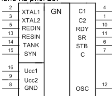
Рис. 25. Условное обозначение ИМС КР580ГФ24
