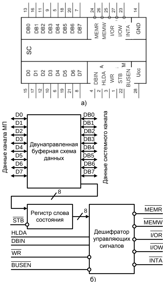
Рис. 76. ИМС системного контроллера КР580ВК28 и КР580ВК38 (а) и их структурная схема (б)
