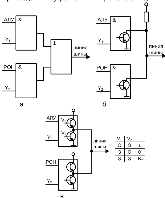
Рис. 5. Подключение нескольких источников к одной шине: а – логическим объединением, б – «монтажным ИЛИ», в – объединением на базе схем с тремя устойчивыми состояниями
