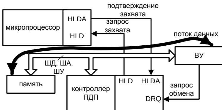
Рис. 69. Организация обмена в режиме ПДП
