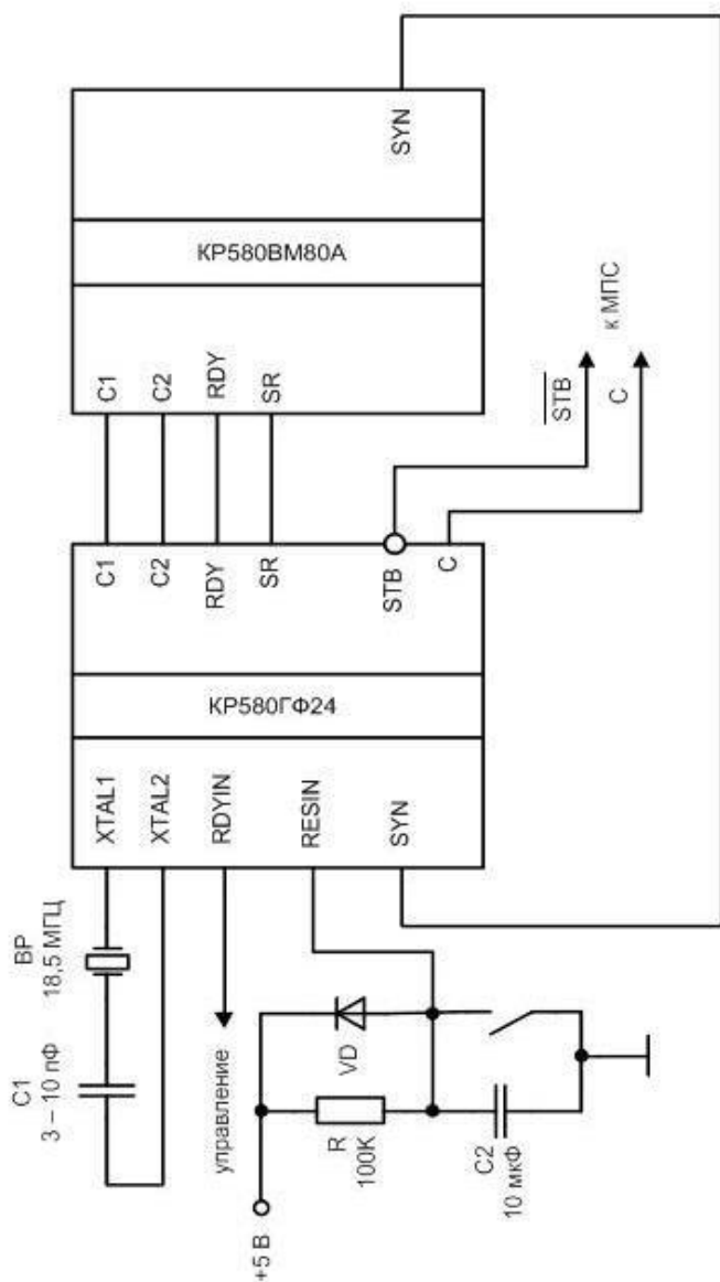
Рис. 23. Схема подключения ИС генератора тактовых импульсов к МП KP580BM80A
