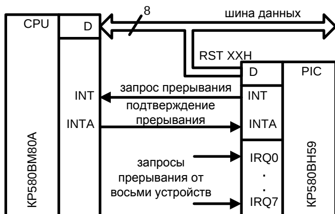
Рис. 68. ИМС контроллера прерываний KP580BH59 (а) и организация ввода/вывода в режиме прерывания
