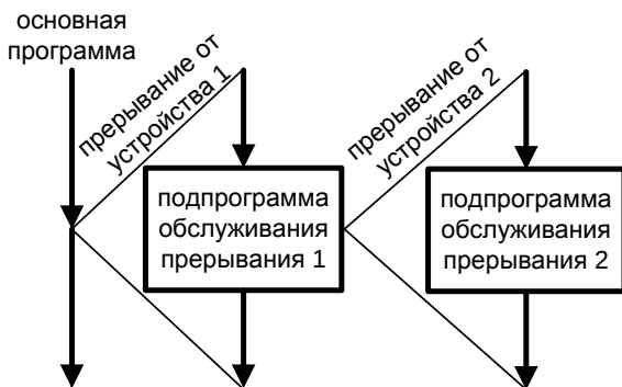
Рис. 65. Многоуровневые (вложенные прерывания)
