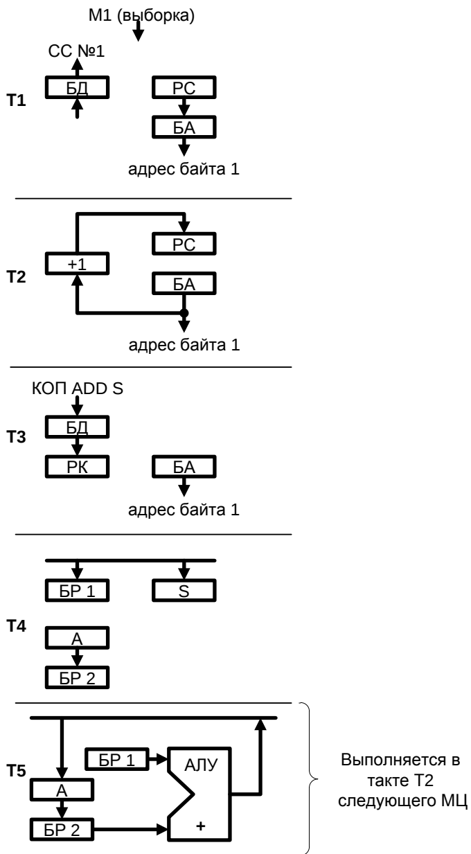
Рис. 60, а. Схема выполнения команд ADD S
