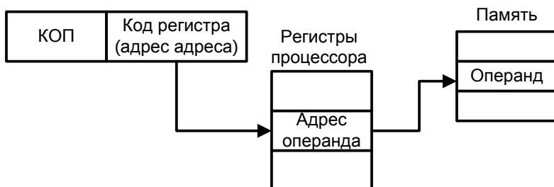
Рис. 15. Косвенная адресация
