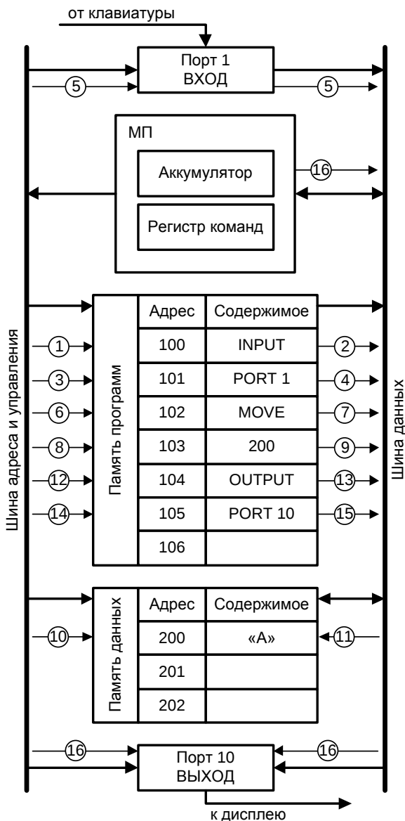
Рис. 8. Диаграмма выполнения процедуры ввода-сохранения-вывода
