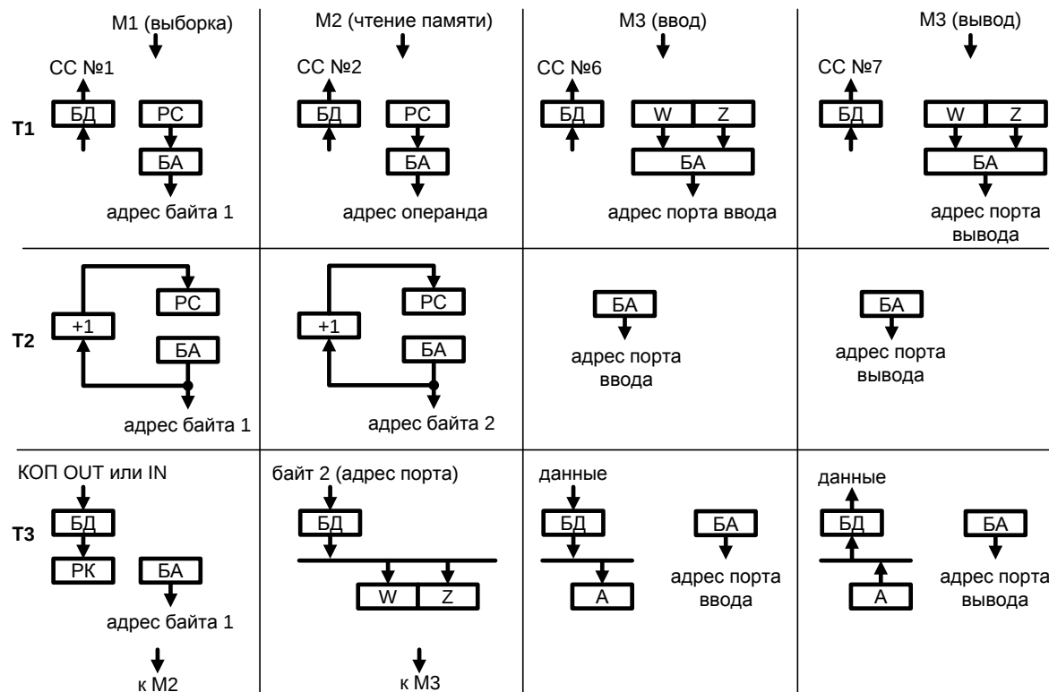
Рис. 60, в. Схема выполнения команд IN / OUT
