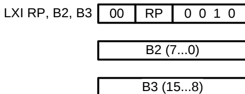
Рис. 46. Формат команд LXI RP, B2, B3
