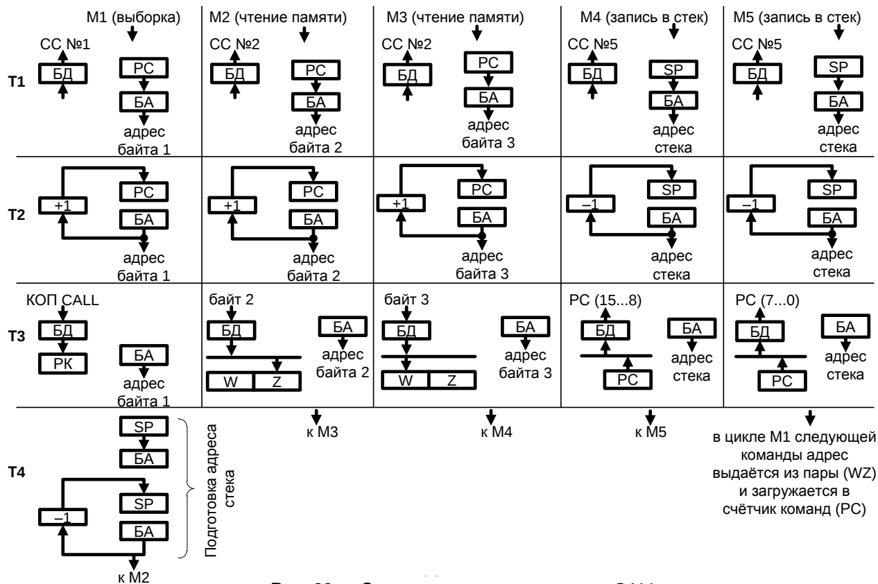
Рис. 60, г. Схема выполнения команды CALL
