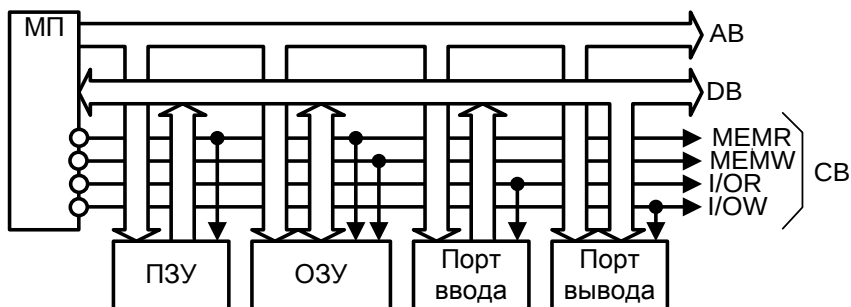
Рис. 6. Структура типичной микроЭВМ
