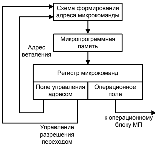
Рис. 10. Функциональная схема блока микропрограммного управления
