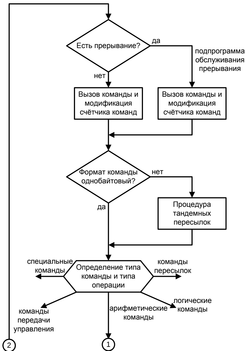
Рис. 58. Рабочий цикл выполнения команды МП КР580ВМ80А (начало)
