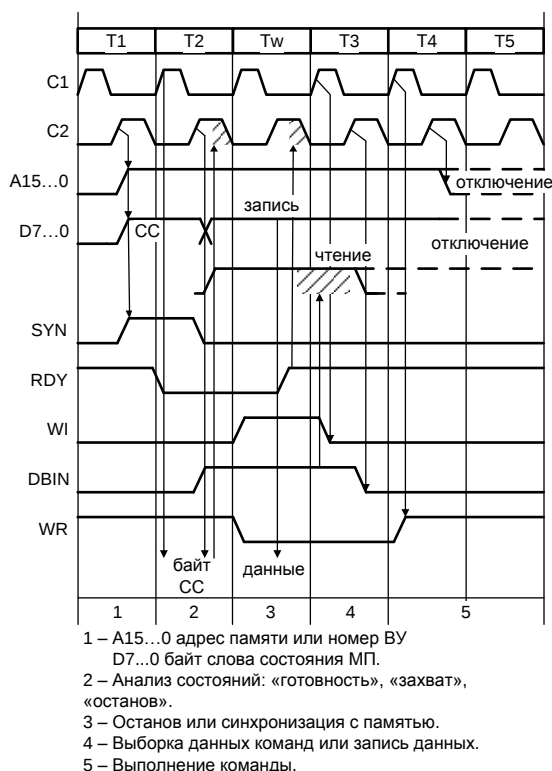
Рис. 61. Временные диаграммы типового машинного цикла МП КР580ВМ80А
