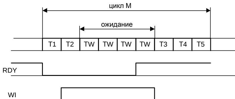
Рис. 63. Формирование режима ожидания МП KP580BM80A
