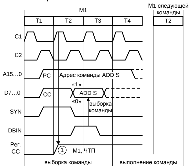
Рис. 62,а. Временные диаграммы выполнения команды ADD S
