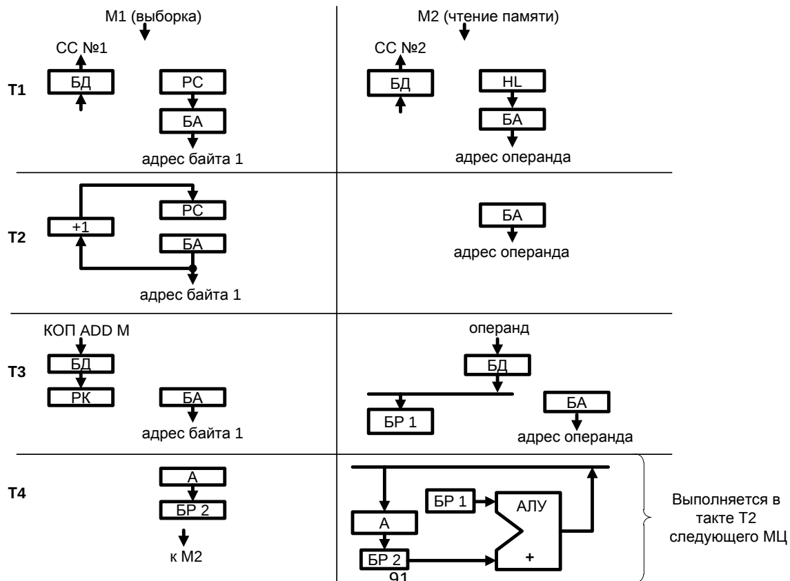
Рис. 60, б. Схема выполнения команды ADD M
