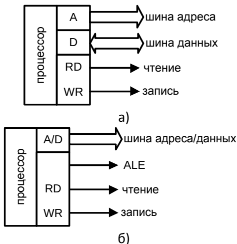
Рис. 4. Микропроцессор: а) с отдельными шинами; б) с совмещёнными шинами
