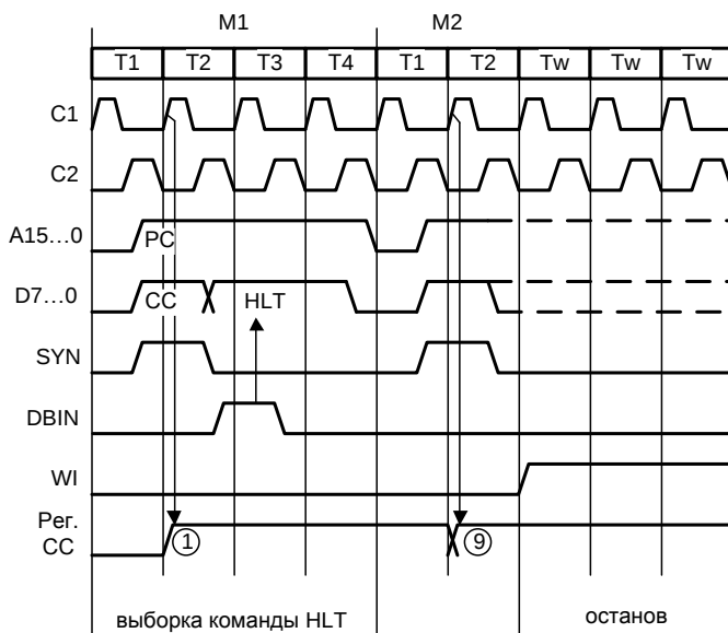
Рис. 72. Временные диаграммы выполнения команды HLT
