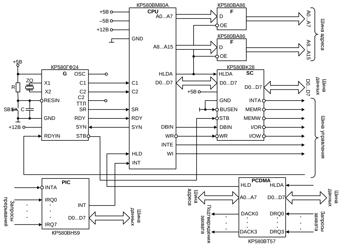
Рис. 77. Микропроцессорный модуль системы на базе МП KP580BM80A
