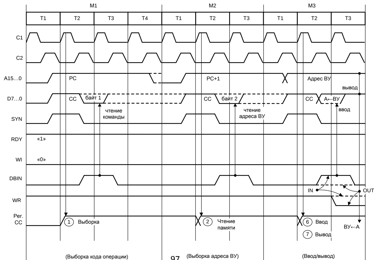
Рис. 62, в. Временные диаграммы выполнения команд IN / OUT
