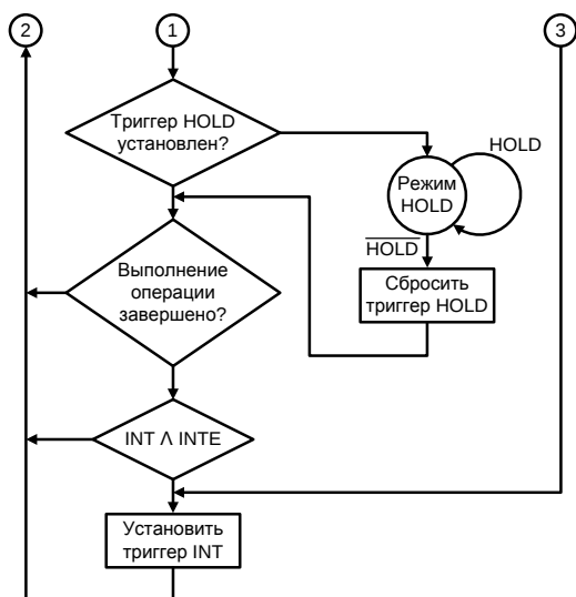
Рис. 59. Алгоритм работы первичного управляющего автомата (окончание)
