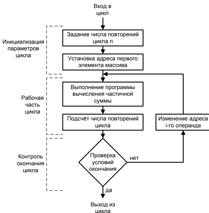
Алгоритм циклической обработки
