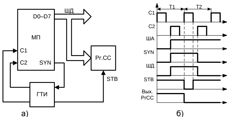
Рис. 57. Фиксация слова состояния микропроцессора
