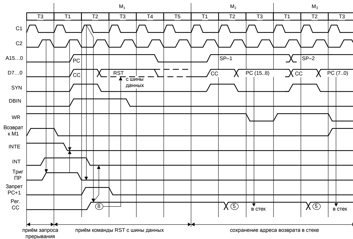
Рис. 67. Схема выполнения (а) и временные диаграммы (б) последовательности перехода в режим прерывания
