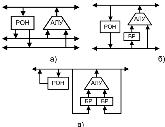
Рис. 3. Топология:
