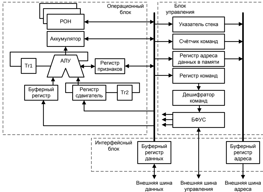
Рис. 9. Типовая структура микропроцессора
