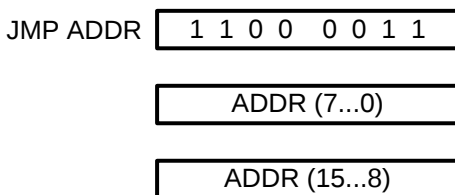
Рис. 40. Формат команды JMP ADDR
