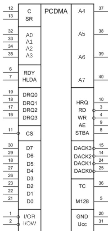
Рис. 71. ИМС контроллера ПДП КР580ВТ57
