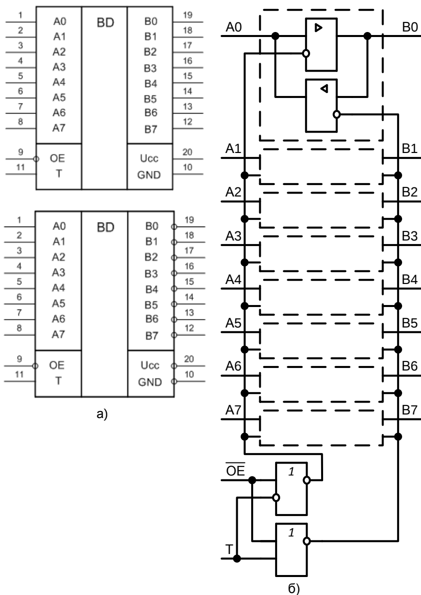
Рис. 75. ИМС шинных формирователей КР580ВА86 и КР580ВА87 (а) и их структурная схема (б)
