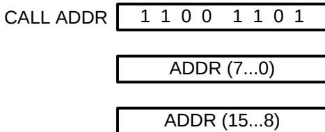
Рис. 41. Формат команды CALL ADDR
