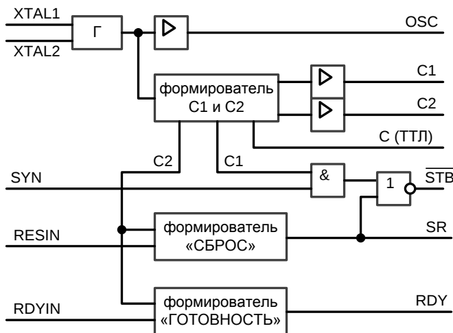
Рис. 22. Функциональная схема генератора тактовых импульсов KP580ГФ24
