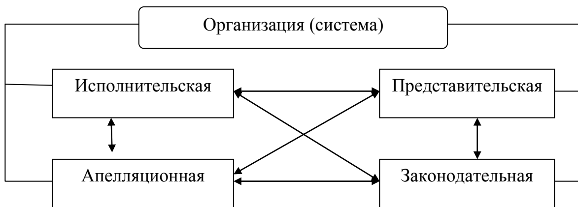
Рис.9. Подсистемы организации [53]
