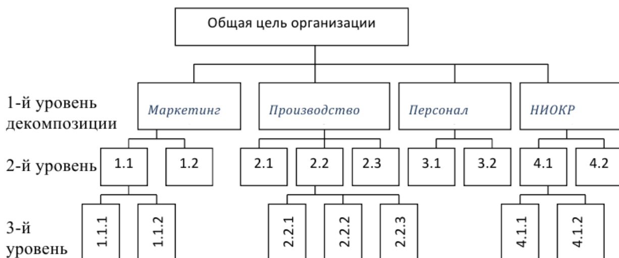
Рис. 16. Дерево целей [27,29]
