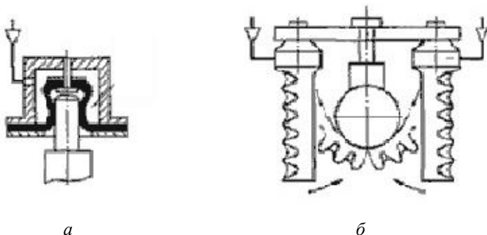
Рис. 1.4. Пневмозахваты
