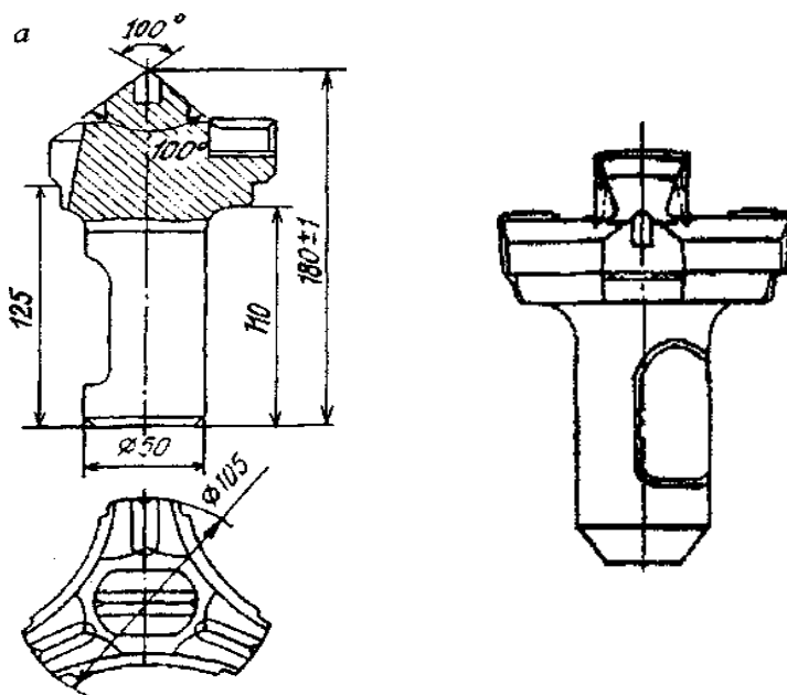
Рис. 3.4. Долото типа К100В
