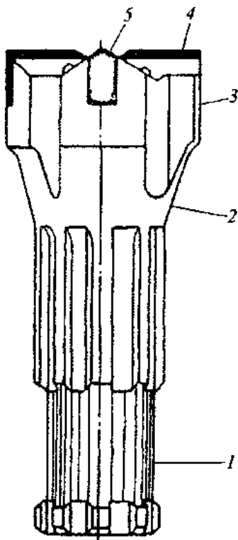
Рис. 3.1. Долото
