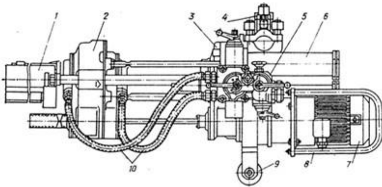
Рис. 1.1. НКР100МА (МВА):
