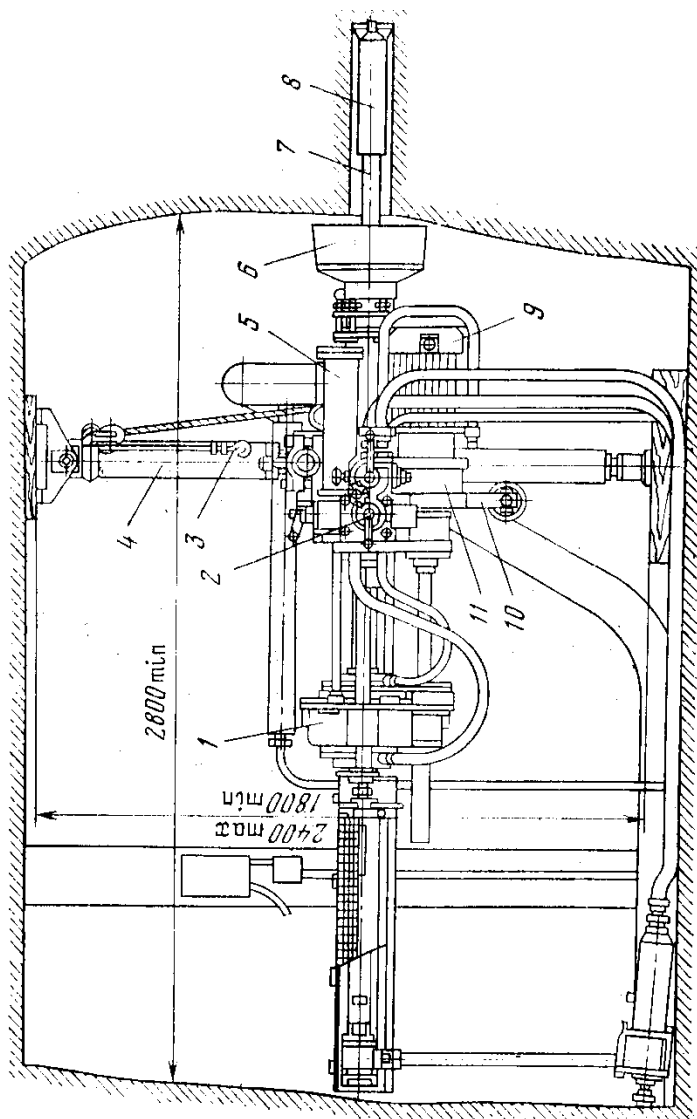
Рис. 1. Буровой станок НКР100МА:
