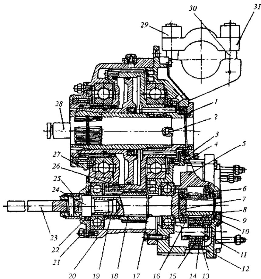
Рис. 1.3. Редуктор с пневмозахватом
