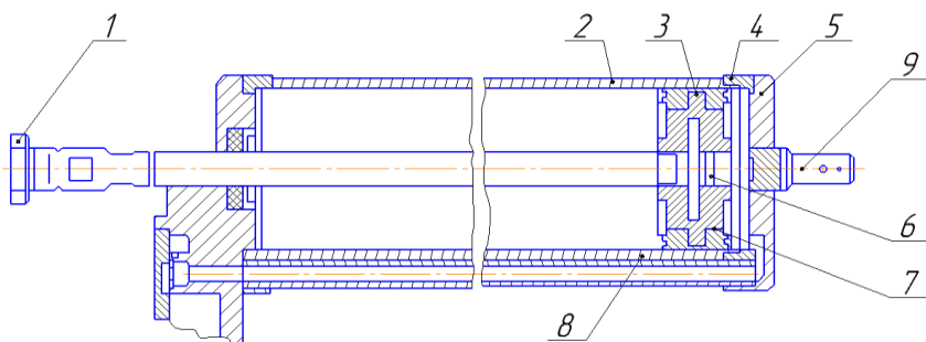
Рис. 2.1. Пневматический податчик
