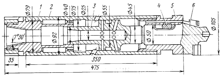
Рис. 3.9. Пневмоударник ПП-105-2,2(П1-75): 1 – переходник; 2 – цилиндр; 3 – ударник; 4 – шпонка; 5 – головка; 6 – долото
