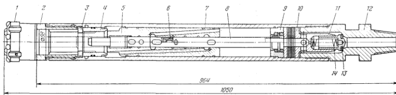
Рис. 3.12. Пневмоударник фирмы «Атлас Копке»: 1 – долото; 2 – букса; 3 – полукольцо; 4 – втулка; 5 – ударник; 6 – перегородка; 7 – цилиндр; 8 – трубка; 9 – ярмо; 10 – крышка; 11 – стакан; 12 – переходник; 13 – обратный клапан; 14 – пружина
