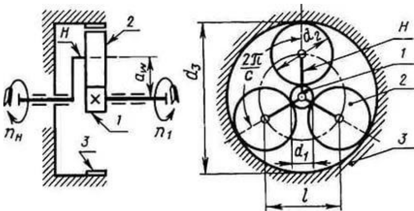
1 – солнечное колесо; 2 – сателлит (планетарная шестерня); 3 – эпицикл (кольцевая шестерня); Н – водило
