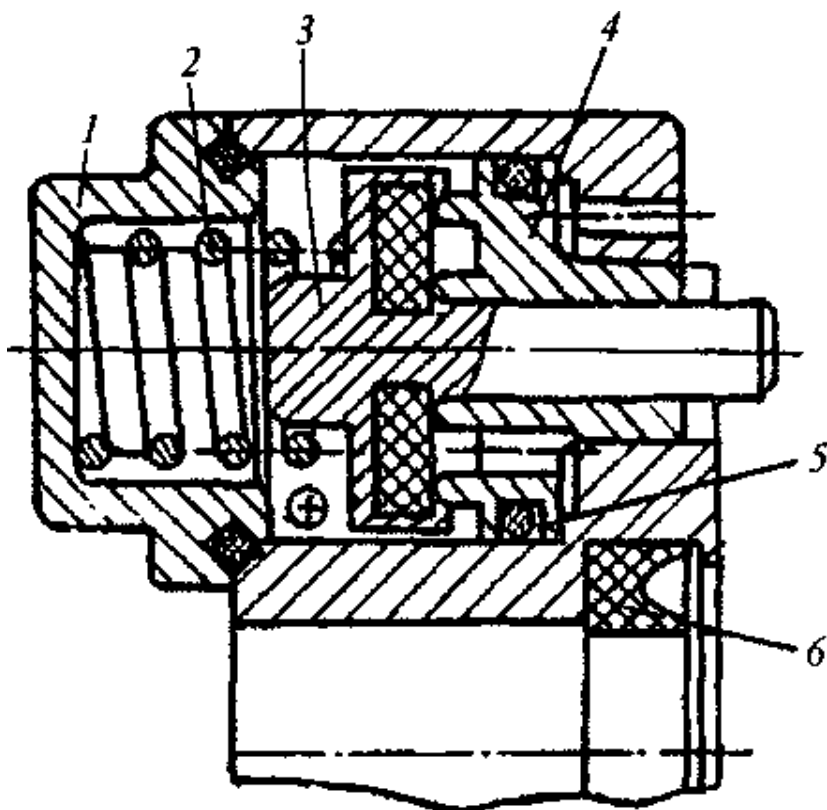
Рис. 2.2. Схема концевого клапана прямого хода
