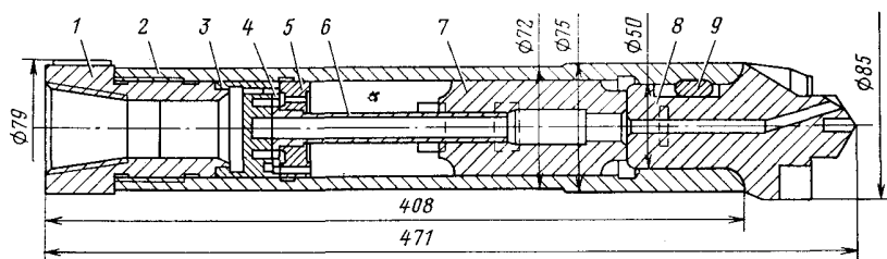
Рис. 3.8. Пневмоударник М29Т:
