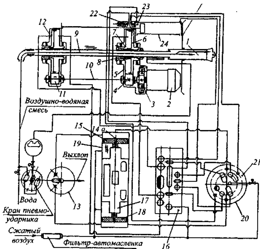
Рис. 2. Принципиальная схема бурового станка НКР-100М
