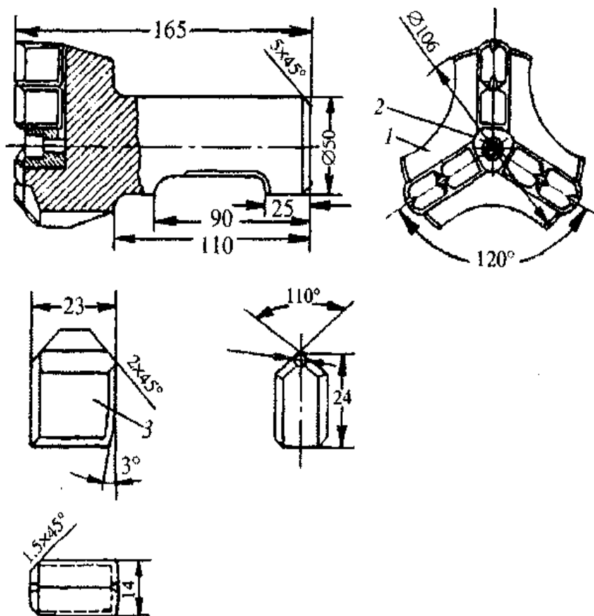
Рис. 3.5. Долото Т-106 с усиленными пластинками твердого сплава: 1 – корпус; 2 – втулка; 3 – пластинки твердого сплава
