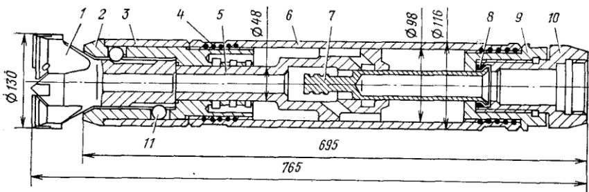
Рис. 3.10. Пневмоударник П125-2,8:
