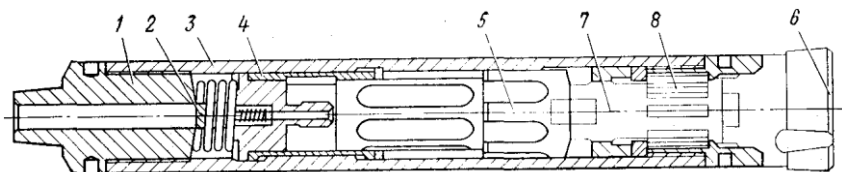
Рис. 3.11. Пневмоударник фирмы «Ингерсол Рэнд», США: 1 – хвостовик; 2 – обратный клапан; 3 – корпус; 4 – гильза; 5 – ударник; 6 – рабочая часть долота; 7 – хвостовик долота; 8 – шлицы на долоте
