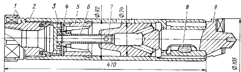
Рис. 3.7. Пневмоударник ПП-105-2,4(М48):
