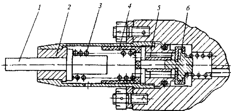
Рис. 2.3. Схема концевой клапана обратного хода
