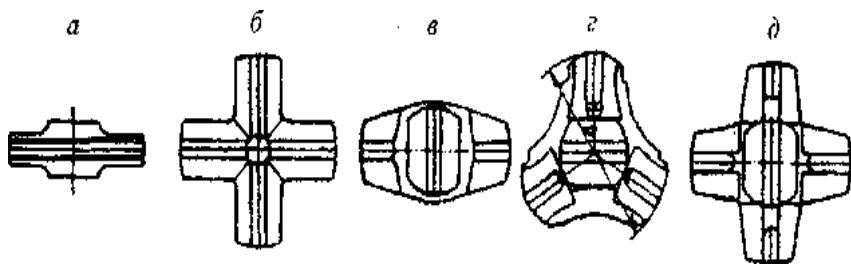
Рис. 3.3. Виды лезвий
