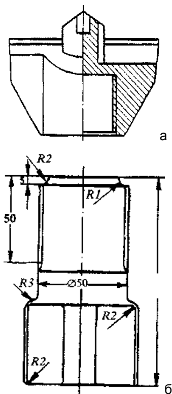
Рис. 3.2. Разъемное долото
